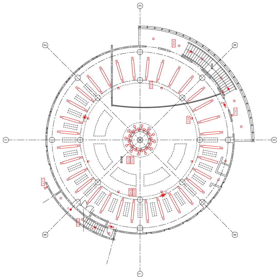
図書館棟 2階平面図 S-1:1/100
