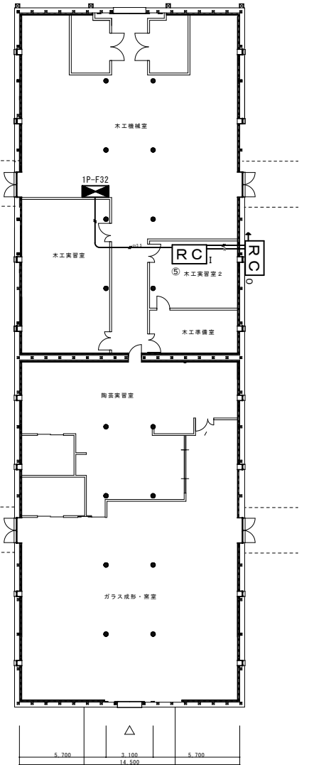
実習棟C. 1階平面図 1/125
