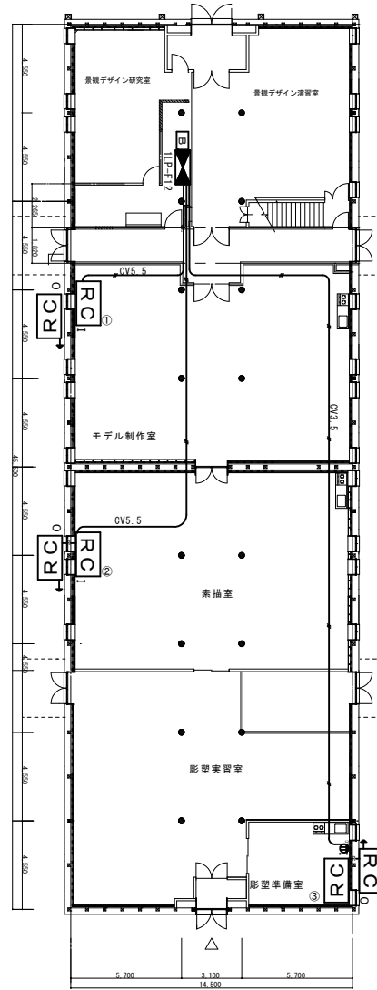
実習棟A. 1階平面図 1/125
